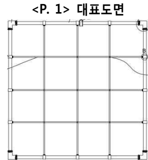
<P. 1> 대표도면 [양식장의 패류 먹이 침강장치를 나타낸 평면도]
